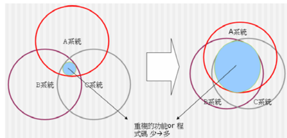
圖 2：重用概念圖[17]
