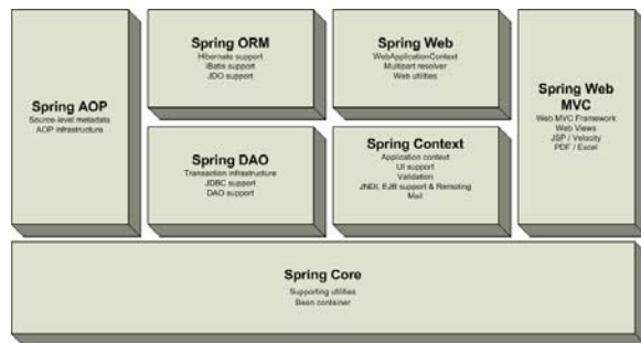
圖 3：Spring 架構圖[17]
