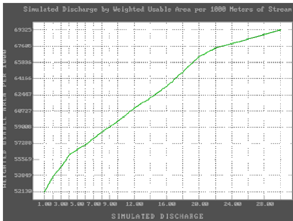
圖10. 流量-WUA關係圖(台灣石魚齒)
