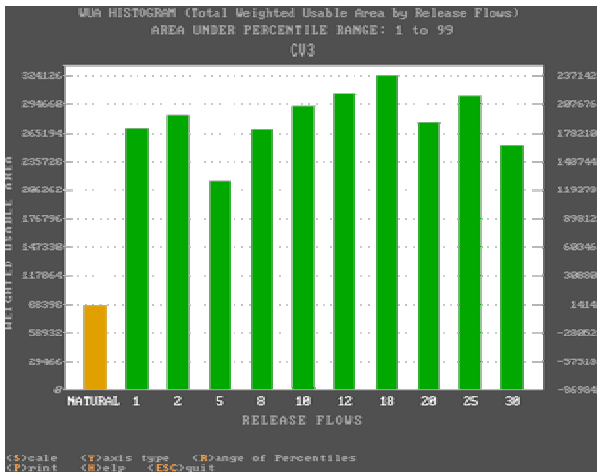
圖 6. 不同生態放流量之 WUA 比較圖 (濁水溪中表層魚類)
