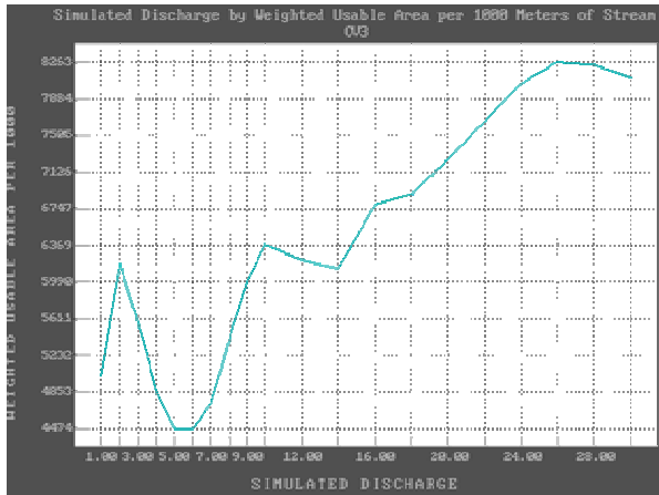
圖9. 流量-WUA關係圖(濁水溪中表層魚類)
