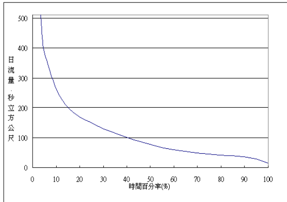
圖4 濁水溪上游日流量延時曲線圖
