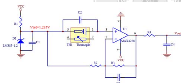
圖4 放大器電路
