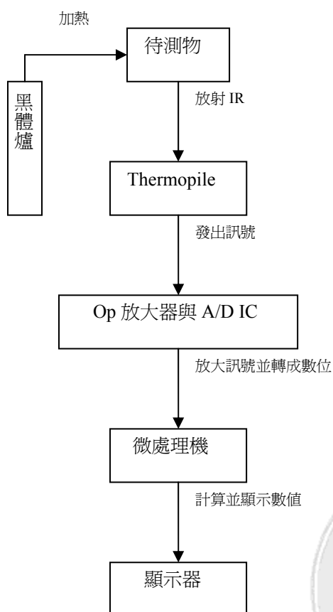
圖6 系統流程圖
